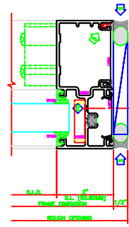
413 RIGHT JAMB 9433
