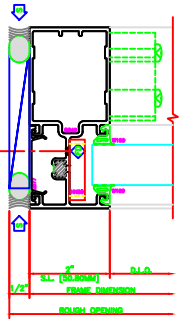
412 LEFT JAMB 9433
