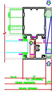
413 RIGHT JAMB 9433
