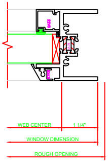
401 JAMB 550G FIXED
